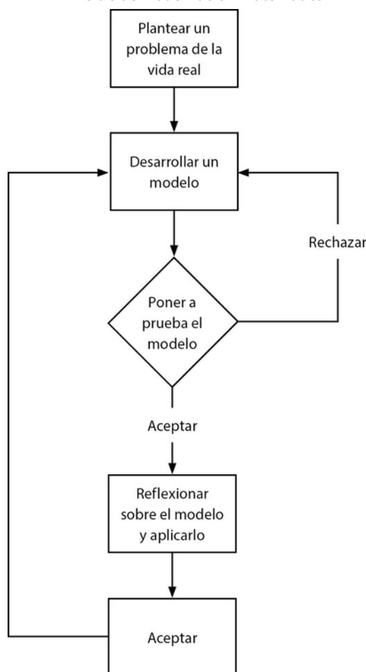
Figura 5 Ciclo de modelización matemática
